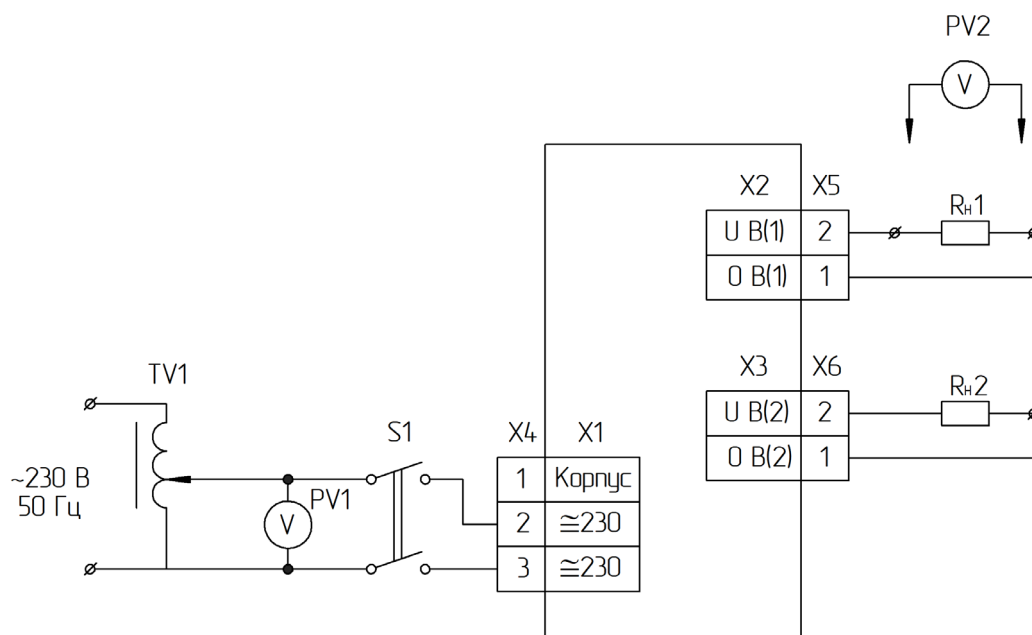
Рисунок 3. Схема для проверки технического состояния модуля питания CP6641
